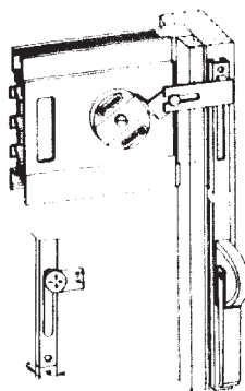
Aufliegendes Gestänge mit Handhebel (Nr. 113) oder Schiebeknopf (Nr. 114)
